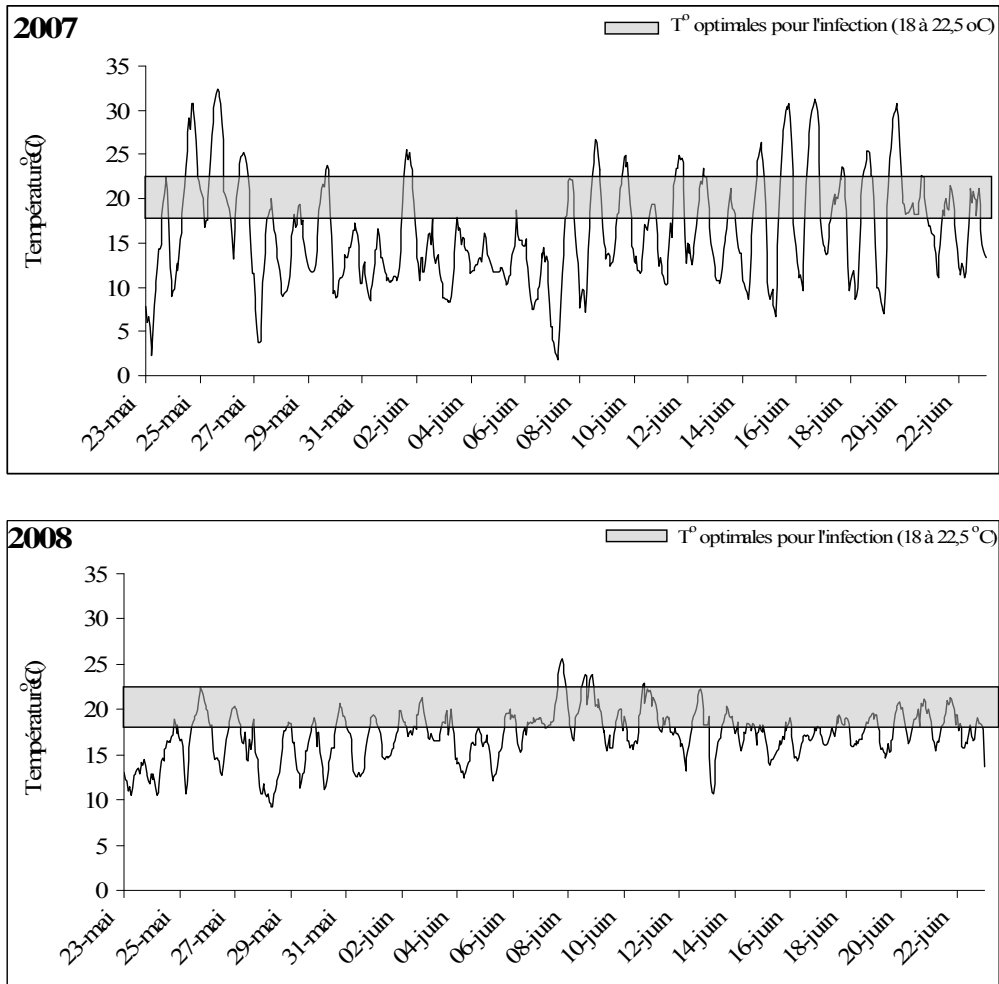
Figure 3. Températures horaires près du couvert végétal dans le fraisier conventionnel (cv Darselect) sur plastique à l'Île d'Orléans.
