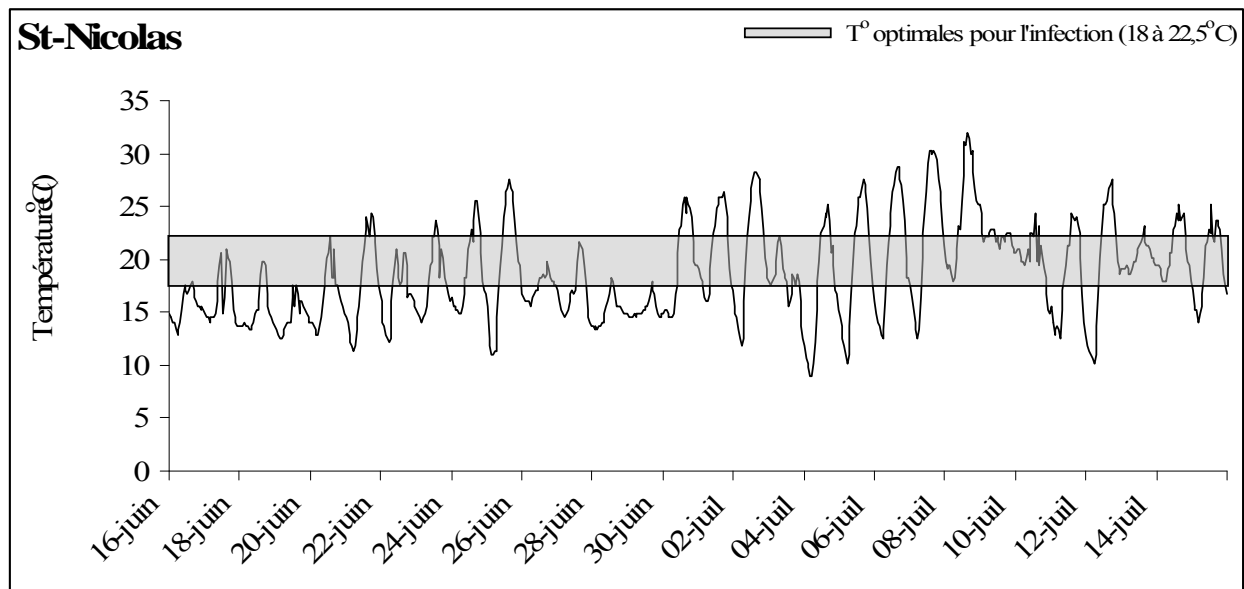
Figure B-5. Températures horaires près du couvert végétal dans le fraisier à jours neutres (cv Seascape), du 16 juin au 15 juillet 2008.
