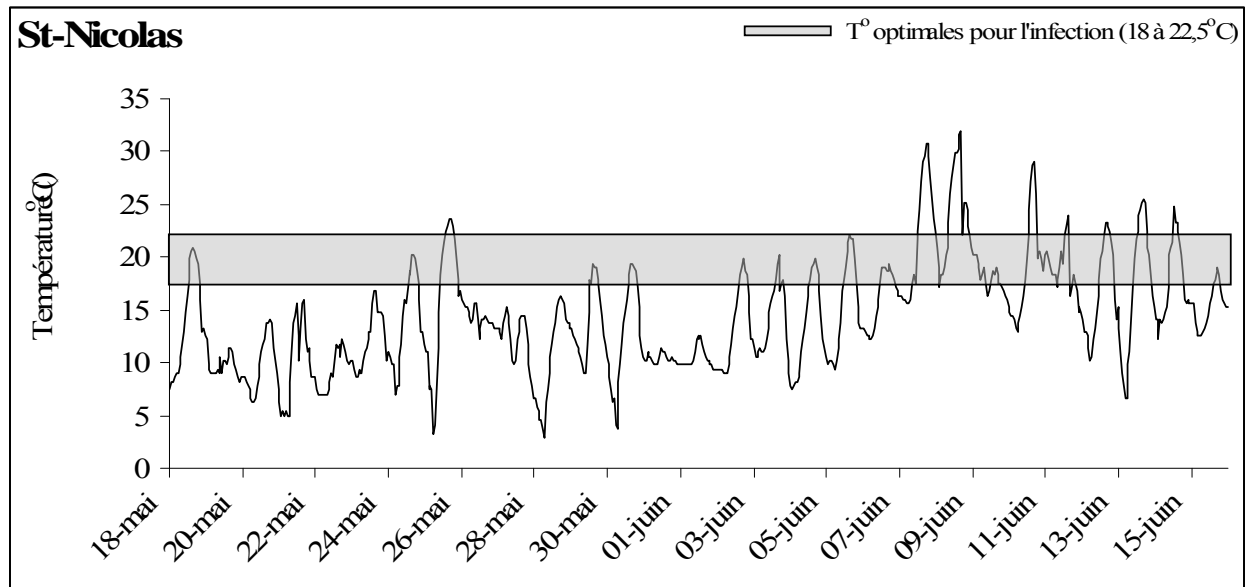
Figure B-4. Températures horaires près du couvert végétal dans le fraisier à jours neutres (cv Seascape), du 18 mai au 15 juin, Île d'Orléans et St-Nicolas, 2008.
