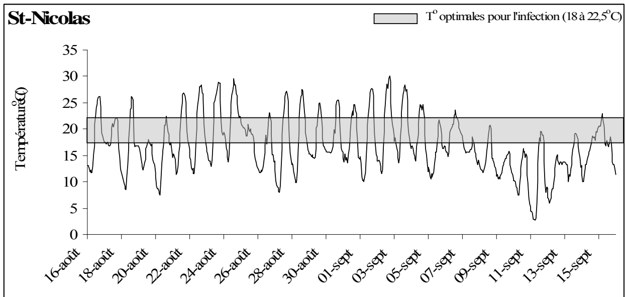
Figure B-7. Températures horaires près du couvert végétal dans le fraisier à jours neutres (cv Seascape), du 16 août au 15 septembre 2008.
